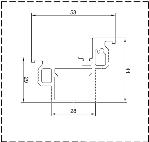
1 SEZIONE PROFILO RASODOOR 53 Rasodoor 53 section
